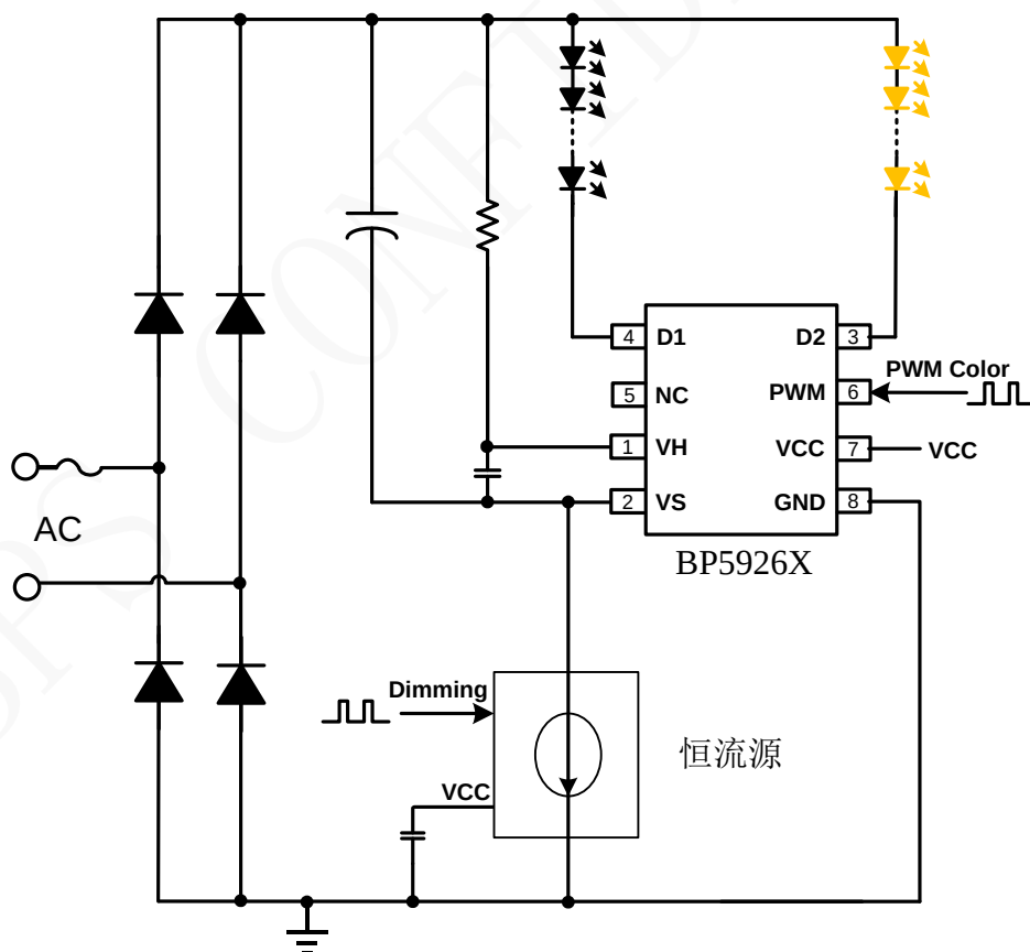
图 1. BP5926X 典型应用图
