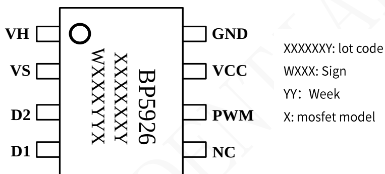
图 2 管脚封装图
