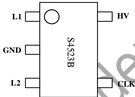
图2 封装脚位图
